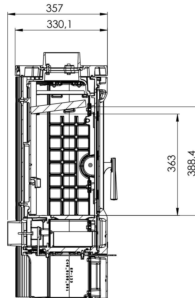
PRZEKRÓJ B-B
