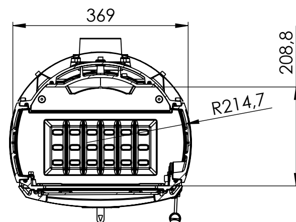
PRZEKRÓJ A-A
