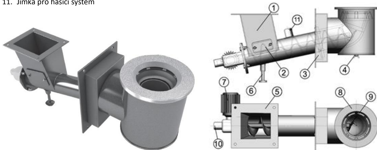
Retortový hořák pro kotle řady H8-A
