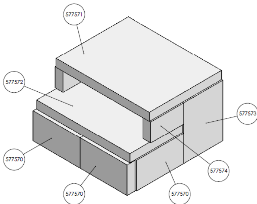
Finální sestava šamotových cihel uvnitř kotle
