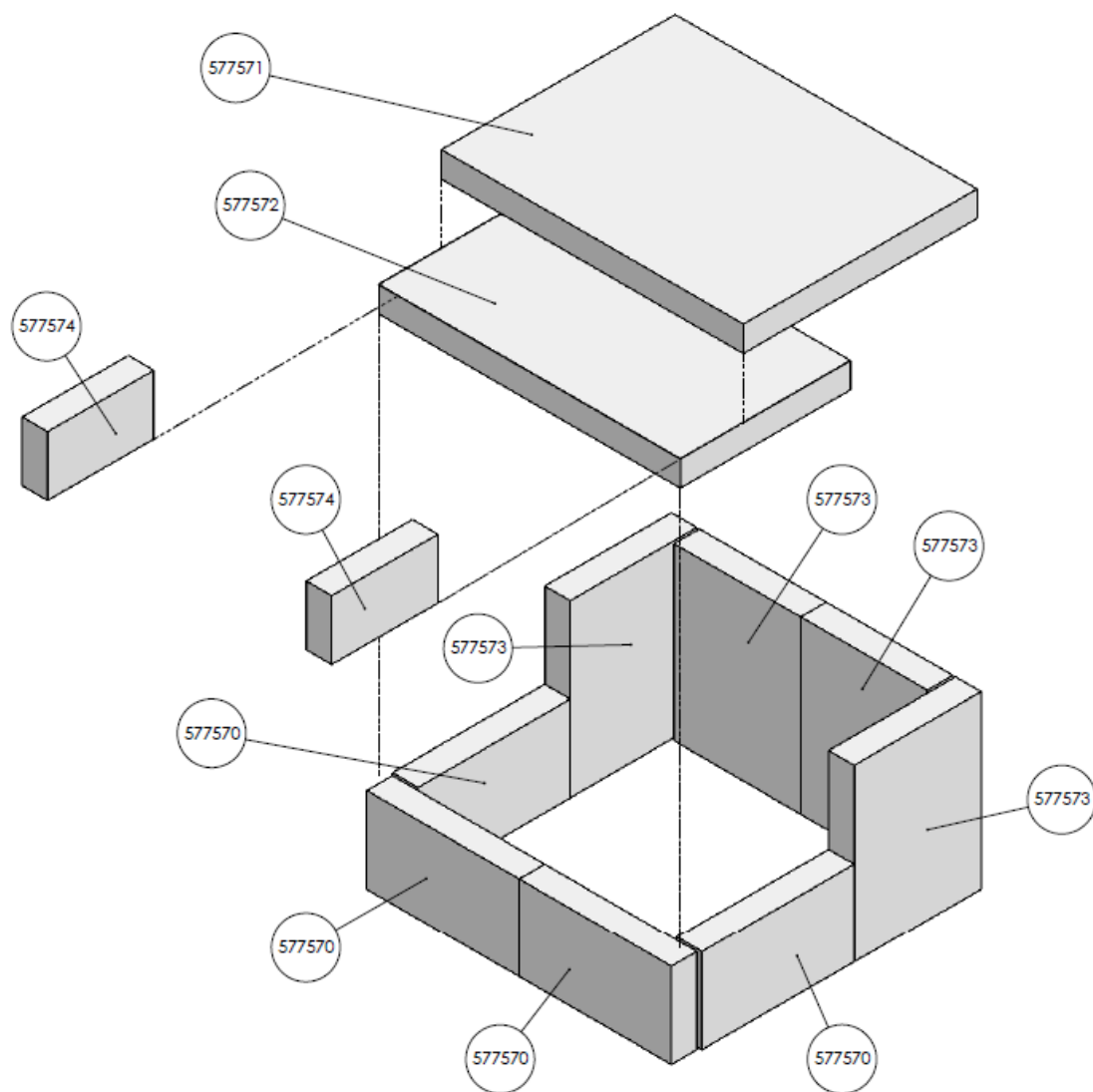
Znázornění postupu instalace šamotových cihel
